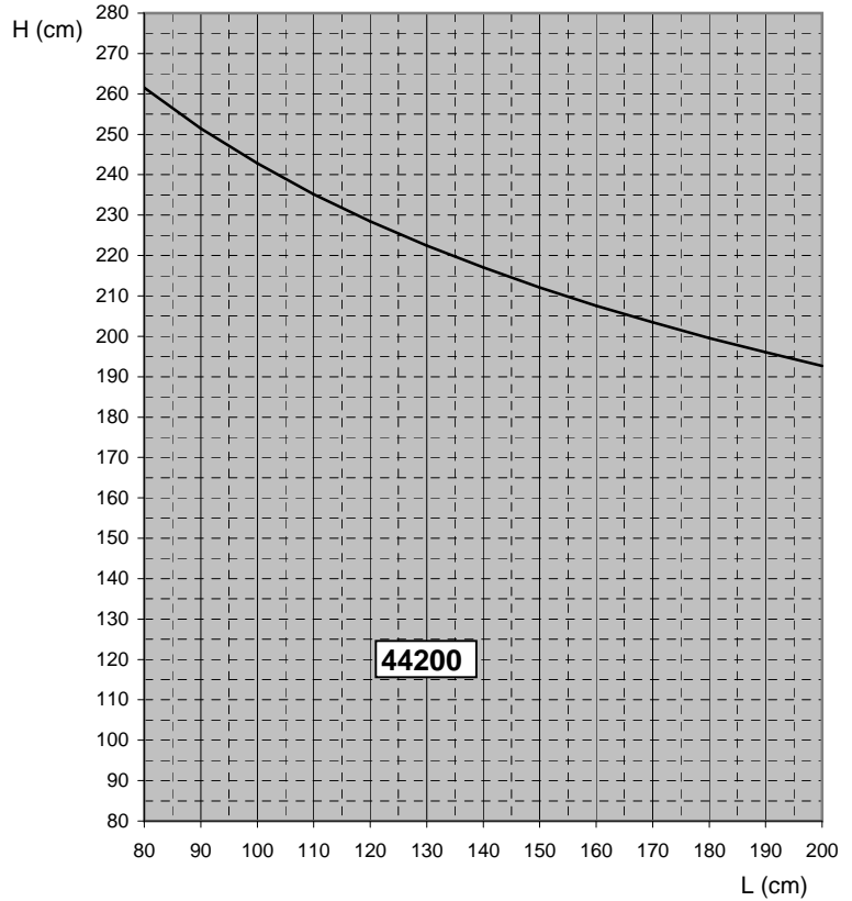
Presión 1000 Pa = 144 Km/h veloc. viento
