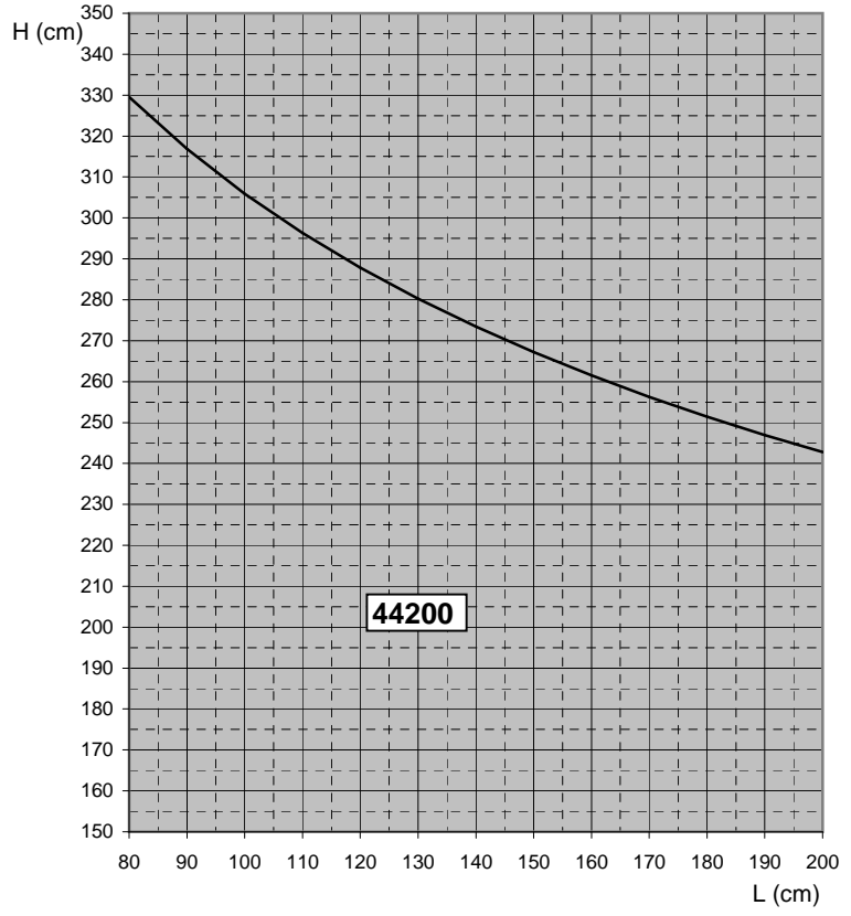
Presión 1000 Pa = 144 Km/h veloc. viento
